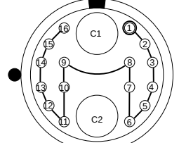
LEMO.EGG.4B.856.ZLL3 KKD16HD Buchse (Lötseite) socket (soldering side)
